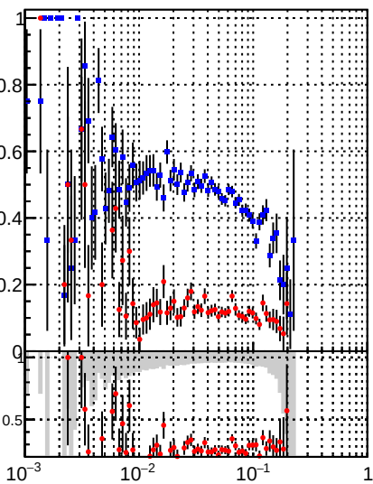
—•— DQM_DisplacedSUSY_mkFit_BDT_ —•— DQM_DisplacedSUSY_mkFit_
