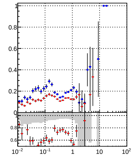
◆ DQM_DisplacedSUSY_mkFit_BDT_ ◆ DQM_DisplacedSUSY_mkFit_
