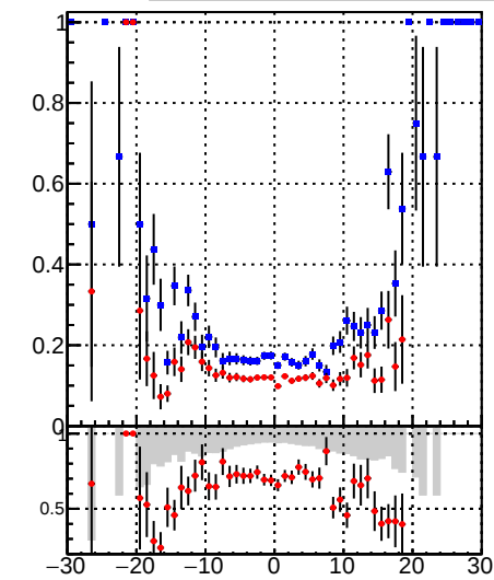
◆ DQM_DisplacedSUSY_mkFit_BDT_ ◆ DQM_DisplacedSUSY_mkFit_
