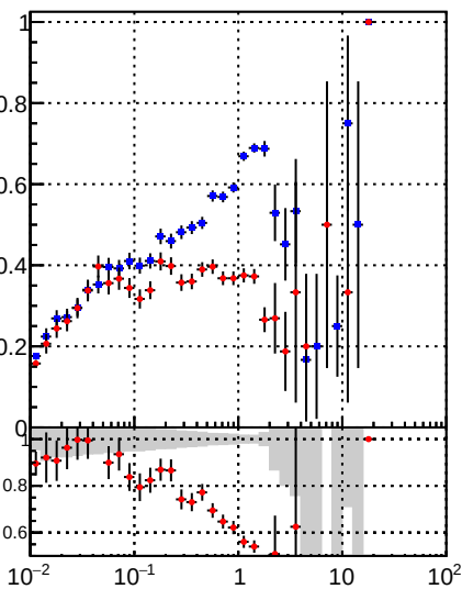
—•— DQM_DisplacedSUSY_mkFit_BDT_ —•— DQM_DisplacedSUSY_mkFit_
