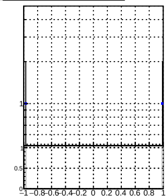
xy(PV)
