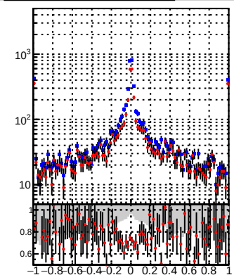
DQM_DisplacedSUSY_mkFit_BDT_ DQM_DisplacedSUSY_mkFit_
