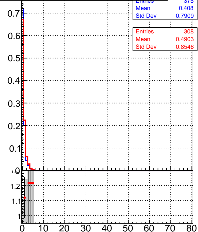
■ DQM_DisplacedSUSY_mkFit_BDT_ ● DQM_DisplacedSUSY_mkFit_
