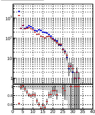
—●— DQM_DisplacedSUSY_mkFit_BDT_ —●— DQM_DisplacedSUSY_mkFit_
