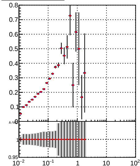
—•— DQM_DisplacedSUSY_mkFit_BDT_ —•— DQM_DisplacedSUSY_mkFit_
