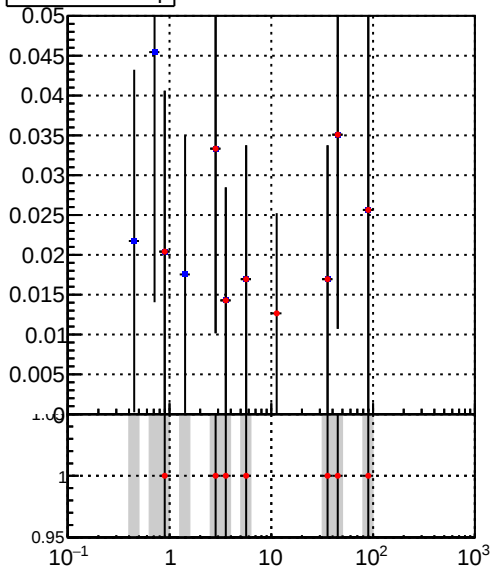
◆ DQM_DisplacedSUSY_mkJit_BDT_ ◆ DQM_DisplacedSUSY_mkJit_
