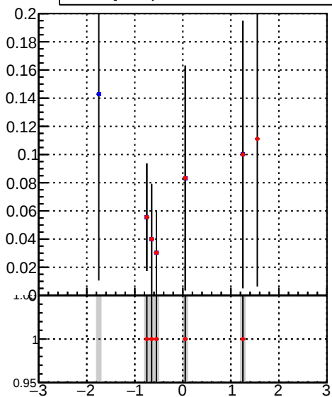
◆ DQM_DisplacedSUSY_mkJit_BDT_ ◆ DQM_DisplacedSUSY_mkJit_
