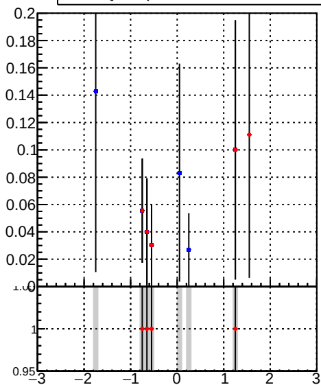
—●— DQM_DisplacedSUSY_mkFit_BDT_ —●— DQM_DisplacedSUSY_mkFit_
