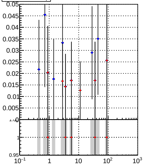
—●— DQM_DisplacedSUSY_mkFit_BDT_ —●— DQM_DisplacedSUSY_mkFit_
