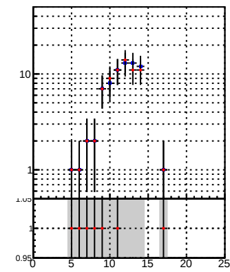
—●— DQM_DisplacedSUSY_mkFit_BDT_ —●— DQM_DisplacedSUSY_mkFit_
