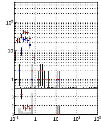
—•— DQM_DisplacedSUSY_mkFit_BDT_ —•— DQM_DisplacedSUSY_mkFit pT eta
