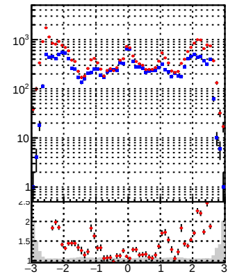
—•— DQM_DisplacedSUSY_mkFit_BDT_ —•— DQM_DisplacedSUSY_mkFit pT eta
