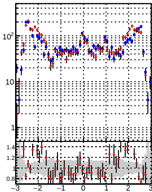
—•— DQM_DisplacedSUSY_mkFit_BDT_ —•— DQM_DisplacedSUSY_mkFit pT eta
