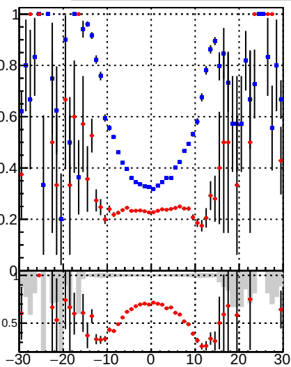
■ DQM_DisplacedSUSY_mkFit_BDT_ ● DQM_DisplacedSUSY_mkFit_
