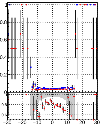
—•— DQM_DisplacedSUSY_mkFit_BDT_ —•— DQM_DisplacedSUSY_mkFit_
