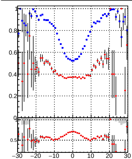
—●— DQM_DisplacedSUSY_mkFit_BDT_ —●— DQM_DisplacedSUSY_mkFit_
