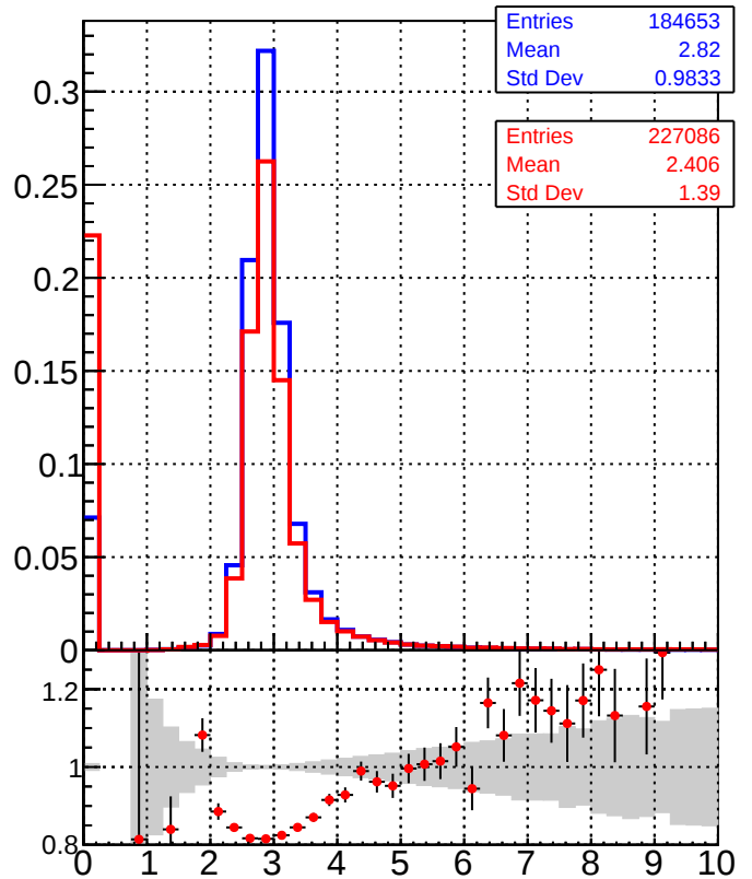
dE/dx estimator 2
