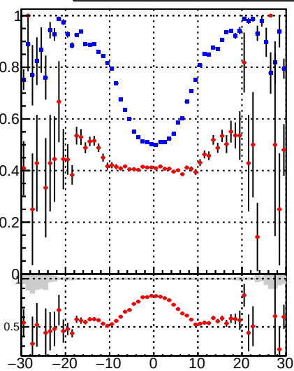
—•— DQM_DisplacedSUSY_mkFit_BDT_ —•— DQM_DisplacedSUSY_mkFit_
