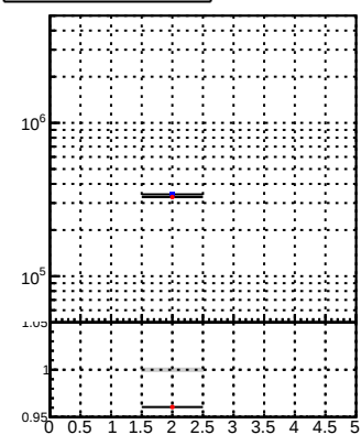
N of reco track vs 3D layer 0 0 1 1 2 2 3 3 4 4 5 5 6 6 7 7 8 8 9 9 10 10 11 11 12 12 13 13 14 14 15 15 16 16 17 17 18 18 19 19 20 20 21 21 22 22 23 23 24 24 25 25 26 26 27 27 28 28 29 29 30 30 31 31 32 32 33 33 34 34 35 35 36 36 37 37 38 38 39 39 40 40 41 41 42 42 43 43 44 44 45 45 46 46 47 47 48 48 49 49 50 50 51 51 52 52 53 53 54 54 55 55 56 56 57 57 58 58 59 59 60 60 61 61 62 62 63 63 64 64 65 65 66 66 67 67 68 68 69 69 70 70 71 71 72 72 73 73 74 74 75 75 76 76 77 77 78 78 79 79 80 80 81 81 82 82 83 83 84 84 85 85 86 86 87 87 88 88 89 89 90 90 91 91 92 92 93 93 94 94 95 95 96 96 97 97 98 98 99 99 100 100
