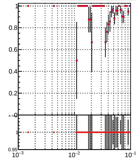
■ DQM_DisplacedSUSY_mkFit_ ● DQM_DisplacedSUSY_mkFit_BDT_
