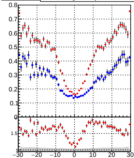
■ DQM_DisplacedSUSY_mkFit_ ■ DQM_DisplacedSUSY_mkFit_BDT_
