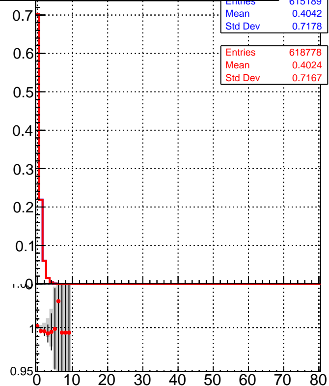
■ DQM_DisplacedSUSY_mkFit_ ● DQM_DisplacedSUSY_mkFit_BDT_
