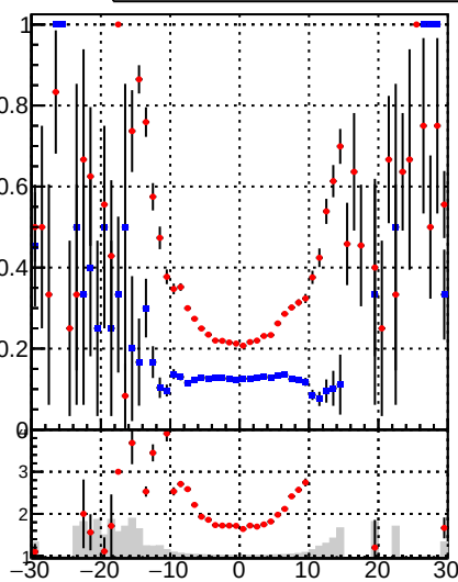
—•— DQM_DisplacedSUSY_mkFit_ —•— DQM_DisplacedSUSY_mkFit_BDT_
