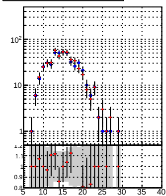
—●— DQM_DisplacedSUSY_mkFit_ —●— DQM_DisplacedSUSY_mkFit_BDT_
