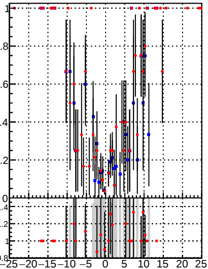
DQM_DisplacedSUSY_mkFit DQM_DisplacedSUSY_mkFit_BDT
