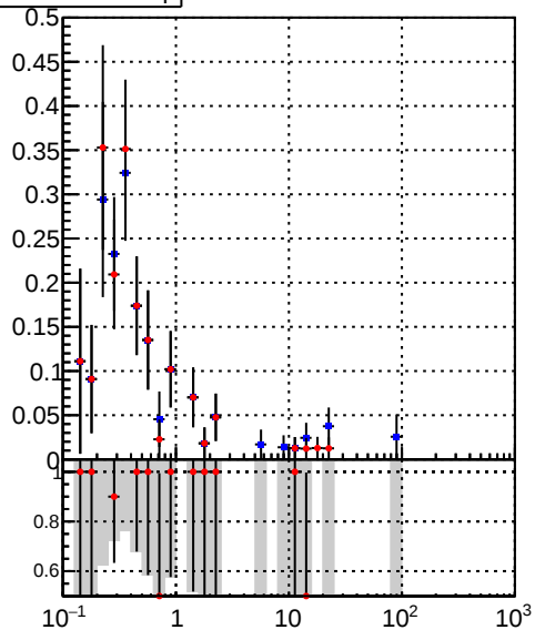
—●— DQM_DisplacedSUSY_mkFit_ —●— DQM_DisplacedSUSY_mkFit_BDT_
