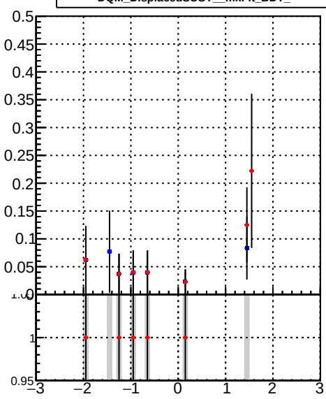
■ DQM_DisplacedSUSY_mkFit_ ■ DQM_DisplacedSUSY_mkFit_BDT_
