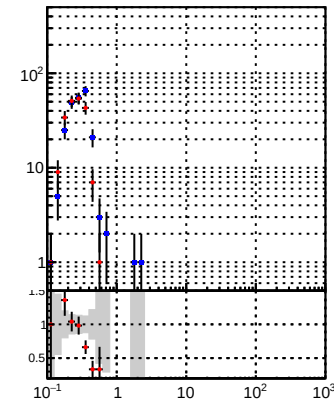
Legend: - DQM_DisplacedSUSY_mkFit (blue circles) - DQM_DisplacedSUSY_mkFit_BDT (red circles) - pT eta
