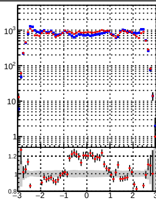
Legend: - DQM_DisplacedSUSY_mkFit (blue circles) - DQM_DisplacedSUSY_mkFit_BDT (red circles) - pT eta
