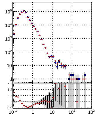
Legend: - DQM_DisplacedSUSY_mkFit (blue circles) - DQM_DisplacedSUSY_mkFit_BDT (red circles) - pT eta
