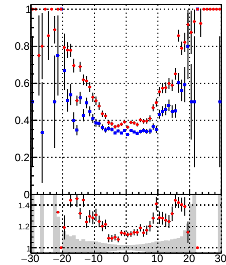
■ DQM_DisplacedSUSY_mkFit_ ■ DQM_DisplacedSUSY_mkFit_BDT_
