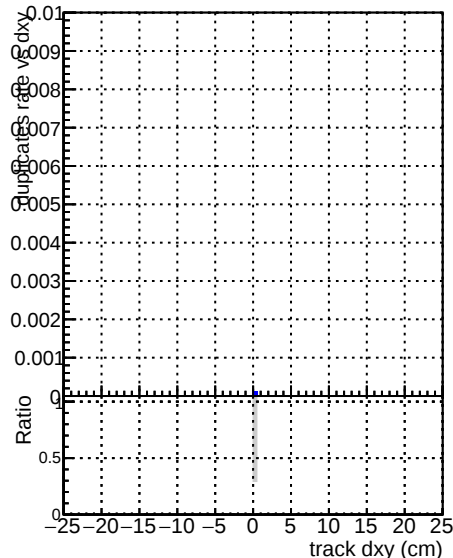
mkFitOriginal OCD RECO a) 0.000 0.000 0.000 a) 0.000 0.000 0.000
