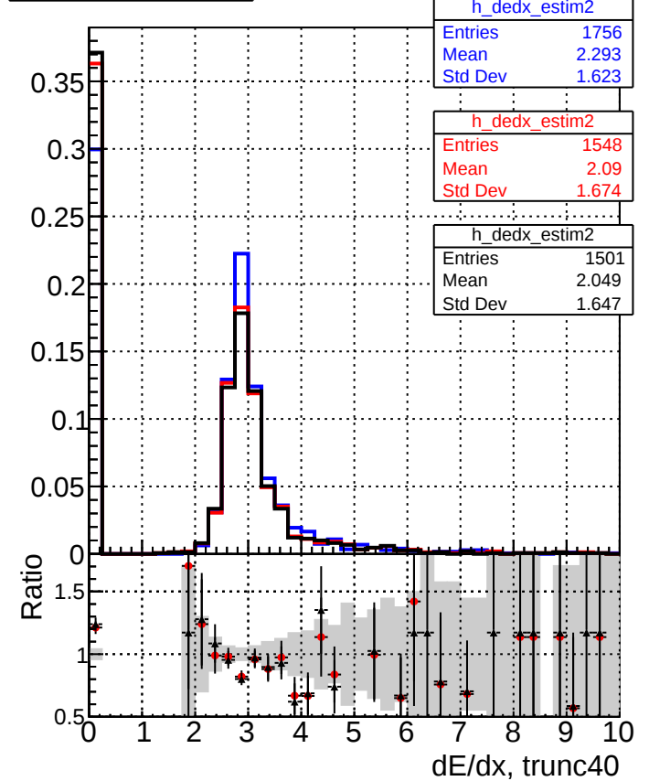
dE/dx estimator 2
