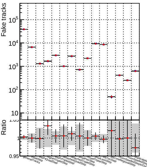
Number —●— DQM_TT_mkFit_MODIF
