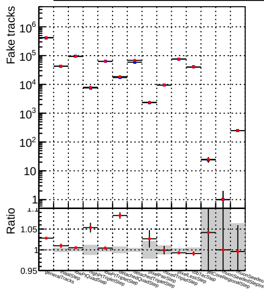
Number —●— DQM_TT_mkFit_MODIF
