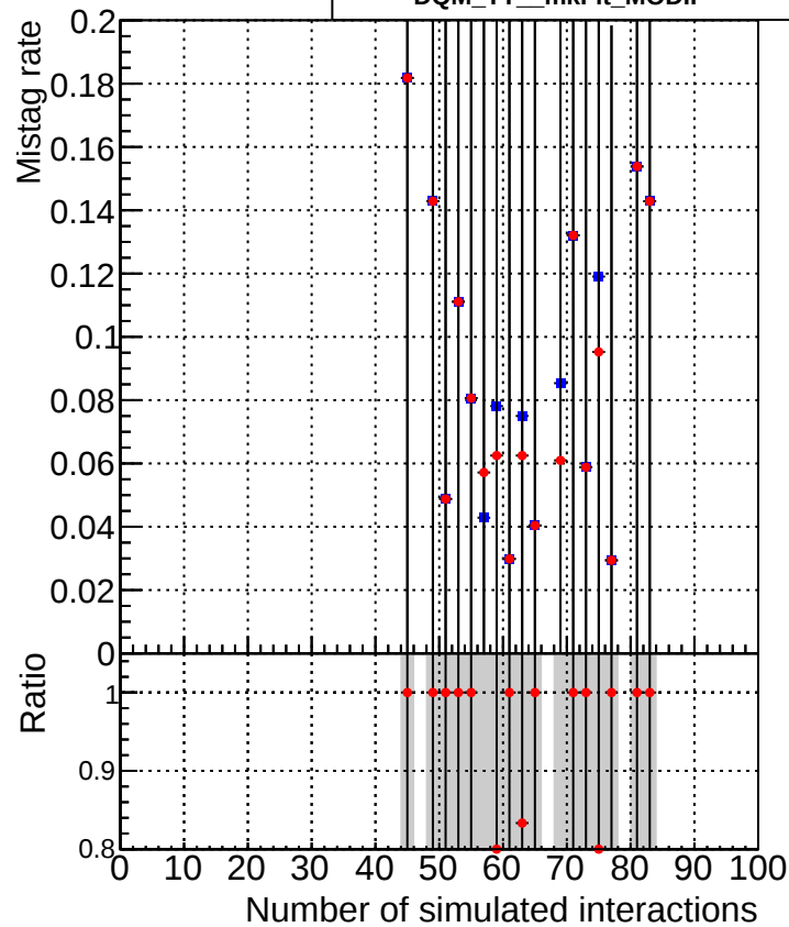
■ DQM_TT_mkFit_ORIG ● DQM_TT_mkFit_MODIF
