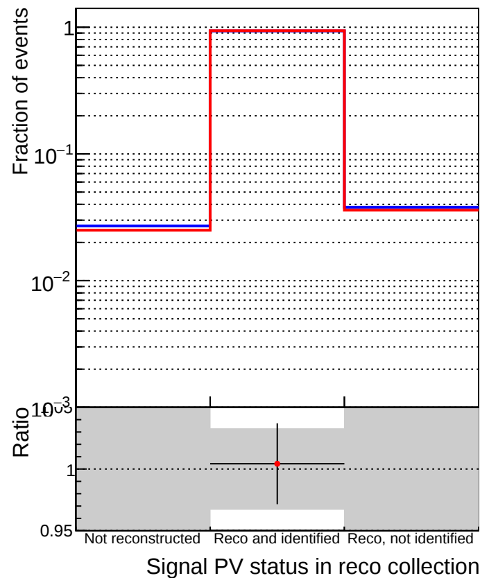
■ DQM_TT_mkFit_ORIG ● DQM_TT_mkFit_MODIF
