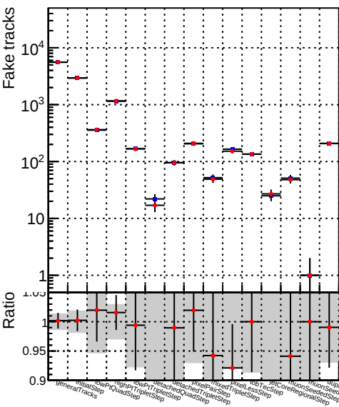
Number —●— DQM_TT_mkFit_MODIF
