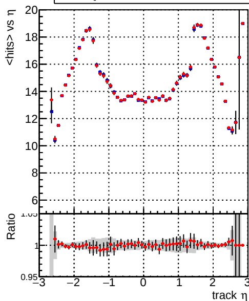
— DQM_TT_mkFit_ORIG — DQM_TT_mkFit_MODIF
