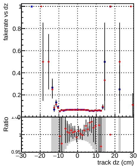
Fake rate vs dz —●— DQM TT mkFit_ORIG —●— DQM TT mkFit_MODIF
