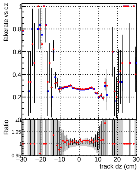
—●— DQM TT mkFit_ORIG —●— DQM TT mkFit_MODIF
