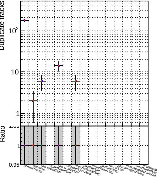
Number DQM V0001 R0000000001 Global mkFitBADINNER RECO DQM V0001 R0000000001 Global mkFitBADOUTER RECO DQM V0001 R0000000001 Global mkFitNOMEAS RECO
