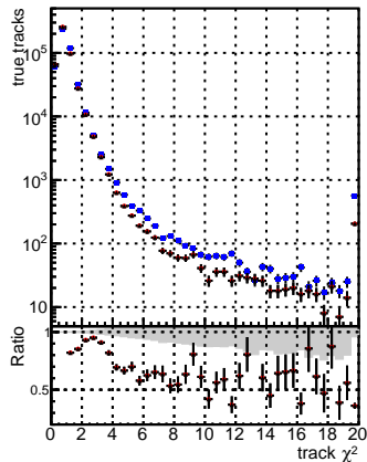
1--Goba--mkFitNewOLD1000time--RECO 1--Goba--mkFitOLD-checkDet--RECO
