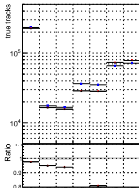
1--Goba--mkFitNewOLD1000time--RECO 1--Goba--mkFitOLD-checkDet--RECO
