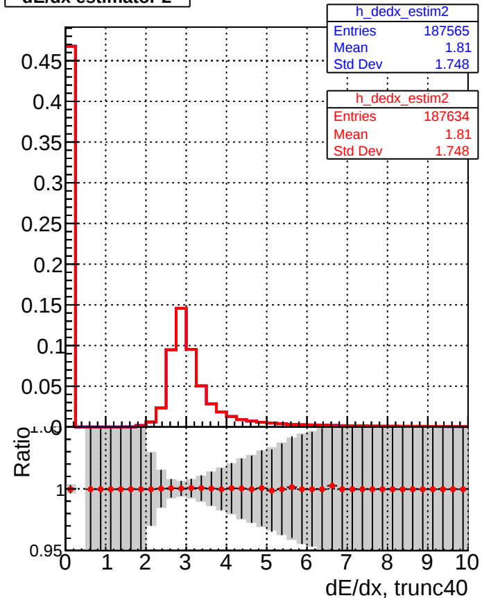
dE/dx estimator 2
