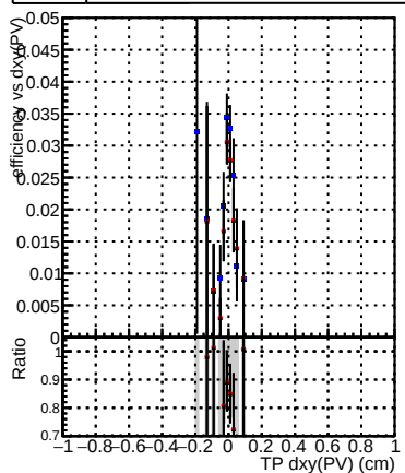
Efficienc → DQM_V0
