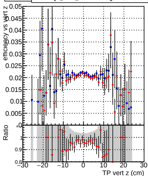
Efficiend —●— DQM_mkFit_TTNEWnoMS-genMatch-CUT
