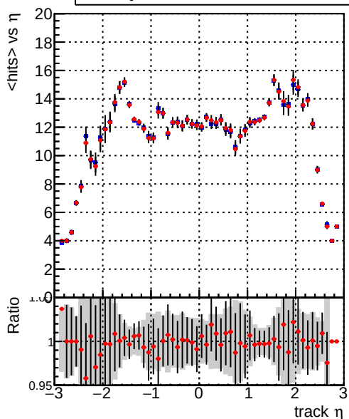
— DQM_mkFit_TToriginal — DQM_mkFit_TTNEUHS_ALLITERS
