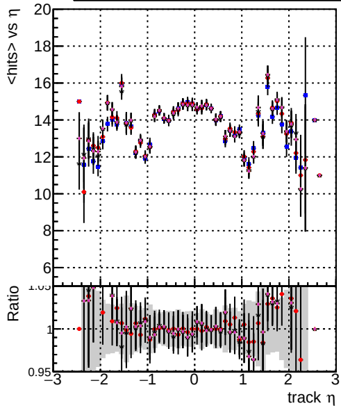
mean hit DQM mkFit TToriginal-106 DQM mkFit TTNEWHSMS ALLITERS-106 DQM mkFit TTNEWHSMS50 ALLITERS-106 DQM mkFit TTNEWHSMS100 ALLITERS-106
