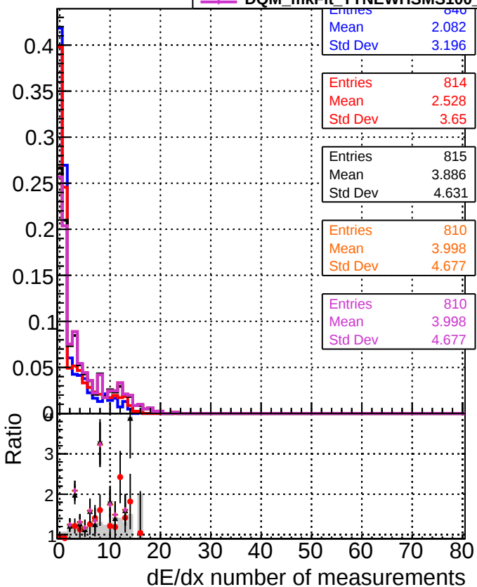
DQM_mkFit TToriginal DQM_mkFit TToriginal-106 DQM_mkFit TTNEWHSMS ALLITERS-106 DQM_mkFit TTNEWHSMS50 ALLITERS-106 DQM_mkFit TTNEWHSMS100 ALLITERS-106
