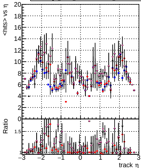
DQM mkFit TToriginal-106 DQM mkFit TTNEWHSMS ALLITERS-106 DQM mkFit TTNEWHSMS50 ALLITERS-106 DQM mkFit TTNEWHSMS100 ALLITERS-106 mean hits
