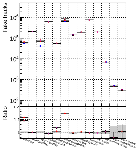
Number —▲— DQM mkFit TTNEWHSMS ALLITERS-106 —+— DQM mkFit TTNEWHSMS50 ALLITERS-106 —*— DQM mkFit TTNEWHSMS100 ALLITERS-106
