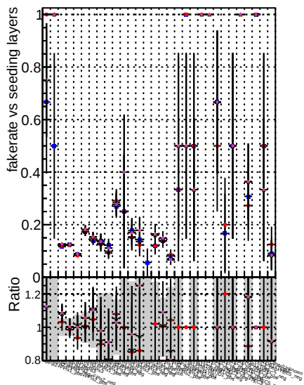
Fake rate vs. DOM mkFit T-iterational+5 ALLTERS-106 DOM mkFit T-iterational+5 ALLTERS-106 DOM mkFit T-iterational+5 ALLTERS-106
