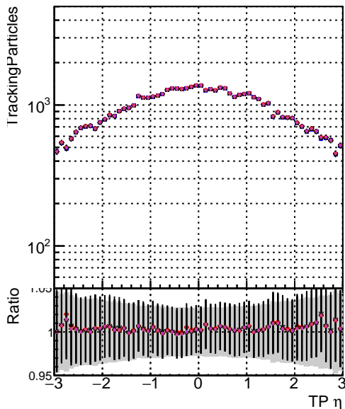
N of sin DQM mkFit TTNEWHSMS95 ALLITERS-106 DQM mkFit TTNEWHSMS50 ALLITERS-106 DQM mkFit TTNEWHSMS100 ALLITERS-106
