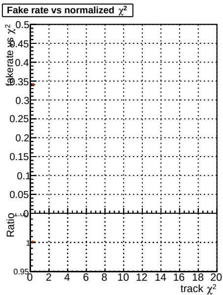
Fake rate vs. —•— BGM mkFit T-Original-106 —•— BGM mkFit T-NEWHSM95-ALLITERS-106 —•— BGM mkFit T-NEWHSM95-ALLITERS-106
