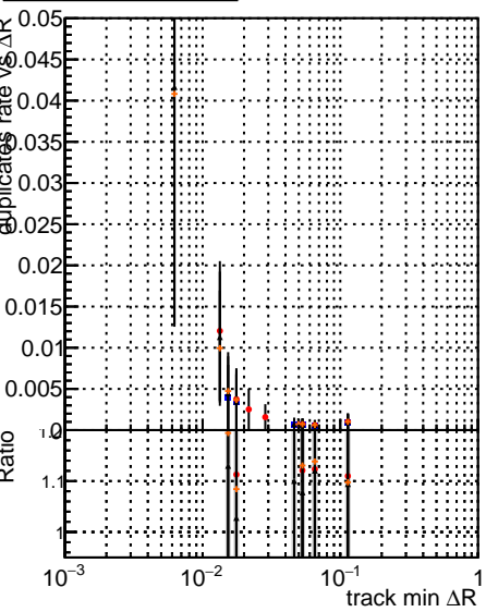
■ DQM mkFit Original ● DQM mkFit Original-106 × DQM mkFit NEWSMS95 ALLITERS-106 × DQM mkFit NEWSMS95 ALLITERS-106
